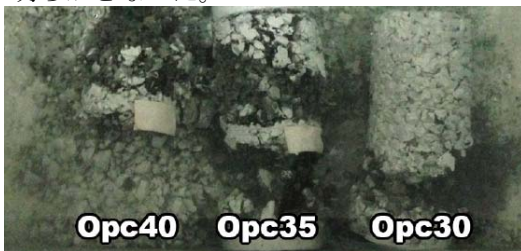
写真-2 塩化カルシウム水溶液に56日間浸漬したポーラスコンクリートの崩壊状況(普通ポルトランドセメント使用、数字はW/Cを示す)
