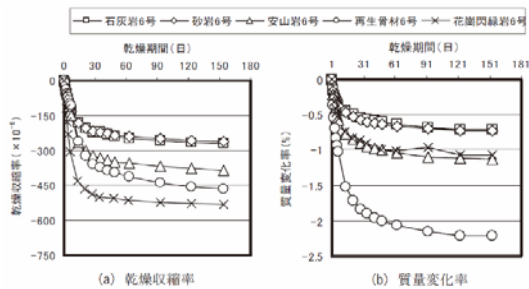
図-9 乾燥収縮率と質量変化率に及ぼす骨材種類の影響
