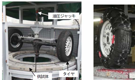
写真-3 回転ラベリング試験装置(左)およびタイヤチェーン(右)
