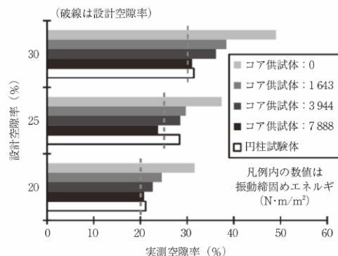
図-4 円柱供試体とコア供試体の空隙率の比較
