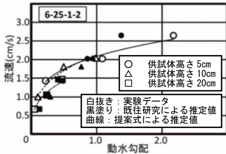
図-6 ポーラスコンクリートの流速と動水勾配の関係の例
