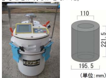
図-5 空隙率測定に用いた広レンジエアメータ(左)およびゴム製アダプタ(右)
