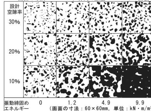
図-2 底面のセメントペーストの垂れの様子（ペーストフロー値：190）
