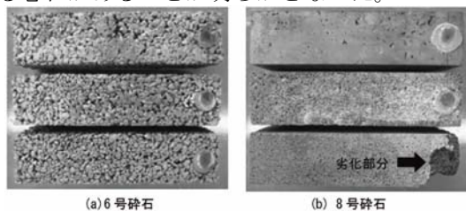
図-10 凍結融解 300 サイクル終了後の供試体の例（設計空隙率：上から10, 20, 30%）
