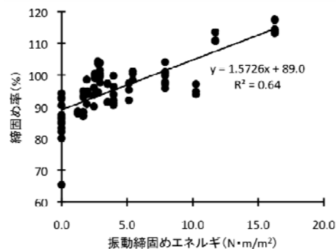
図-1 空隙率/設計空隙率と振動締固めエネルギーの関係
