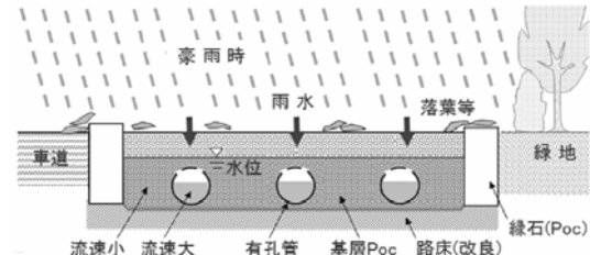
図-11 地盤内で貯水・排水を行う工法の一例（歩道）
