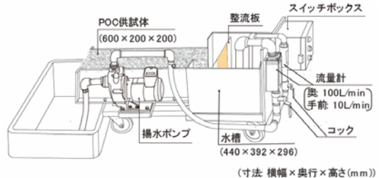
図-12 水平方向透水試験装置
