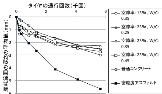
図-8 摩耗深さの平均値とタイヤの通行回数(千回)の関係の例
