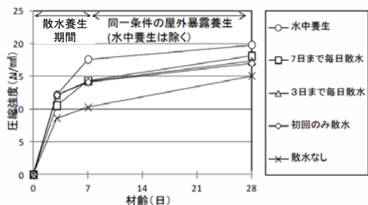
図-3 養生期間が圧縮強度発現に及ぼす影響の例(夏季)
