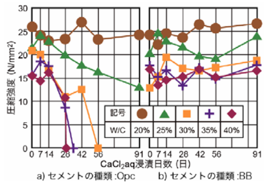
図-7 塩化カルシウム水溶液に浸漬したポーラスコンクリートの圧縮強度の推移 (Opc: 普通ポルトランドセメント、BB: 高炉セメント)
