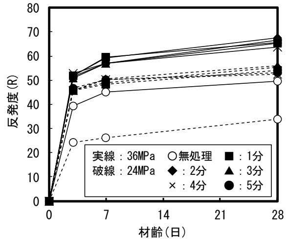
図4 スラブ表面の反発度と材齢の関係
