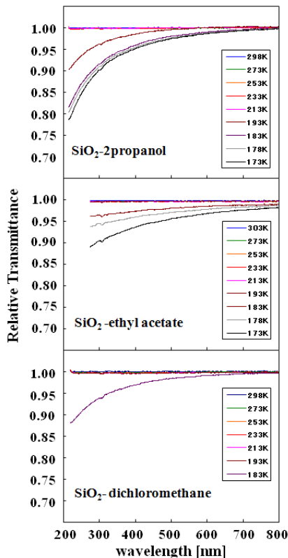
図5：SiO 2 への有機ガス吸着による透過率の変化。色の違いは吸着温度の違いを表す
