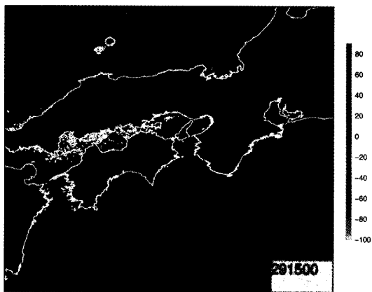
図8 図7と同じ図。ただし、14:00 - 15:00 JSTの図である
