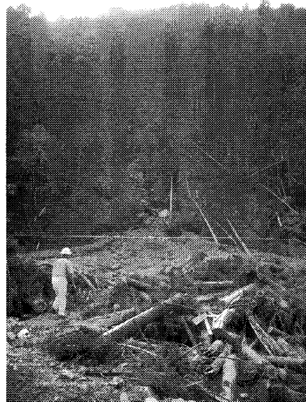
写真5 三軒家地区の斜面崩壊
