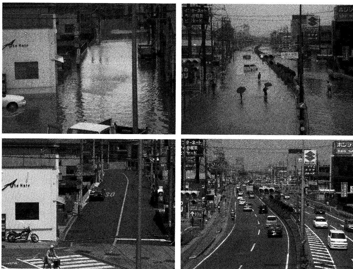
写真1 津市（三重大学近辺）の浸水害。下段の写真は、対応する上段の写真（三重大学小林康之氏撮影）の、平常時の姿
