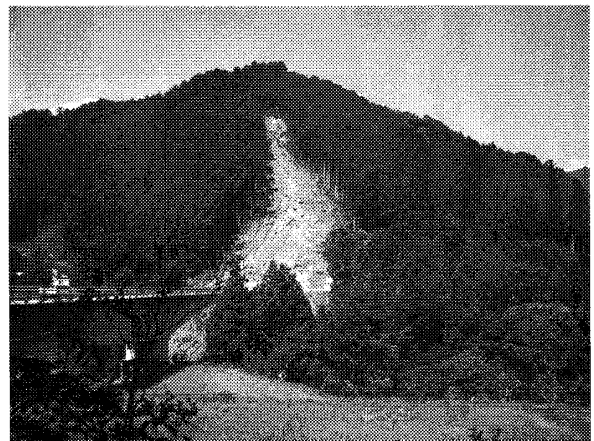
写真2 小滝地区の表層崩壊と土砂流下跡(以下, 場所については, 図10参照)
