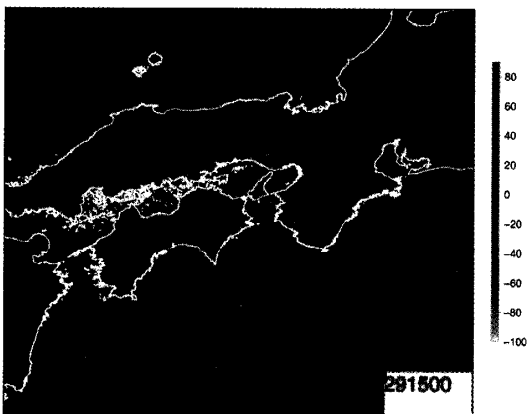
図9 図7と同じ図。ただし、20:00 - 21:00 JSTの図である
