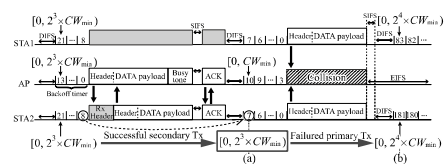
図 6 改良型バックオフ手法
