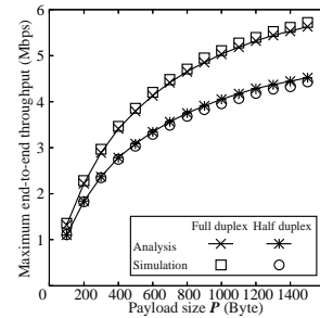
図 3 解析モデルのシミュレーションの結果の比較
