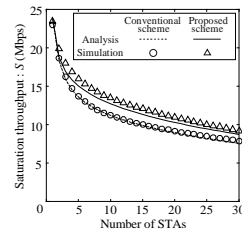
図7 従来型および改良型バックオフ手法における性能比較
