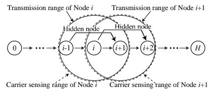
図 2. 無線全二重通信マルチホップネットワーク
