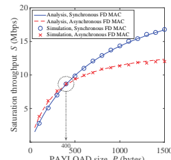
図 5 非同期型および同期型 FD MAC の性能比較
