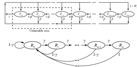
図 4. FD MAC の数理モデルの改良型
