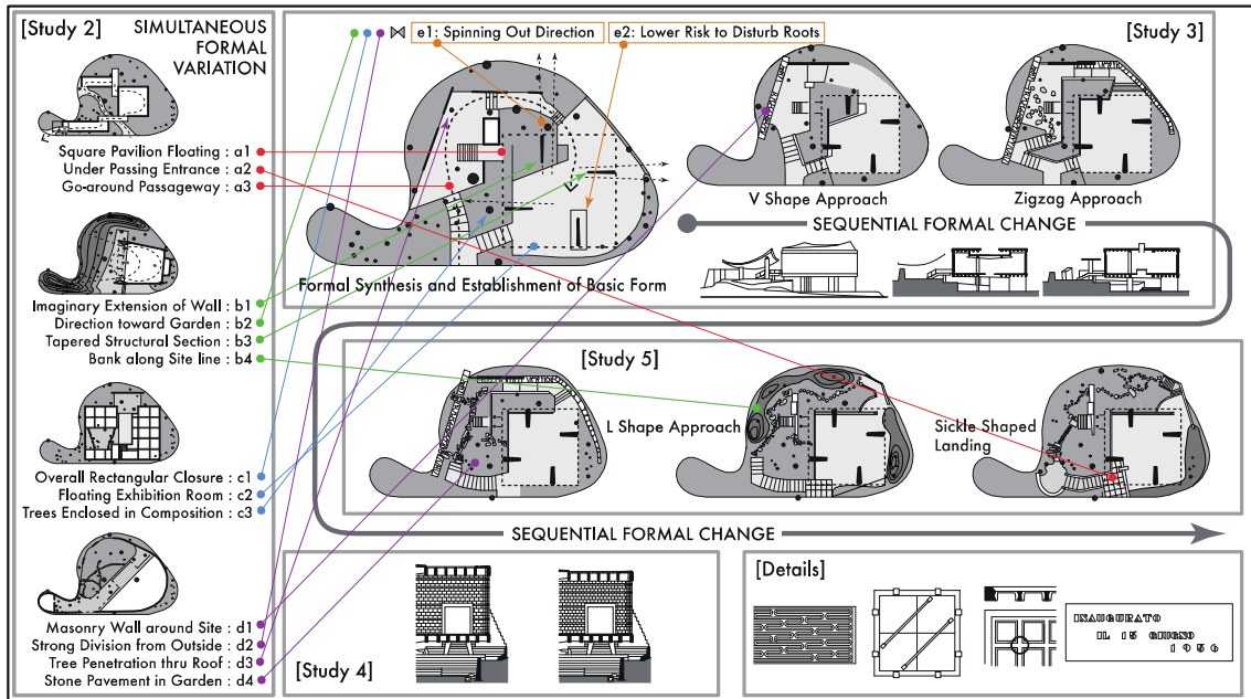
図 3 : 形態分析をもとにした設計過程の問題解決過程 (例), 発表論文から引用, Tomioka Y, Tabata C, Ojika T. Design process of Japanese pavilion in Venice Biennale (1956) by Takamasa Yoshizaka. Jpn Archit Rev. 0000;00:1-15. https://doi.org/10.1002/2475-8876.12305
