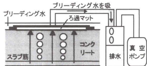
図-1 真空脱水締固め工法の概略図
