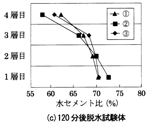
図-10 各位置における水セメント比
