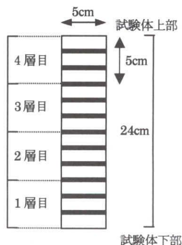
図-4 コア試験体の切断位置
