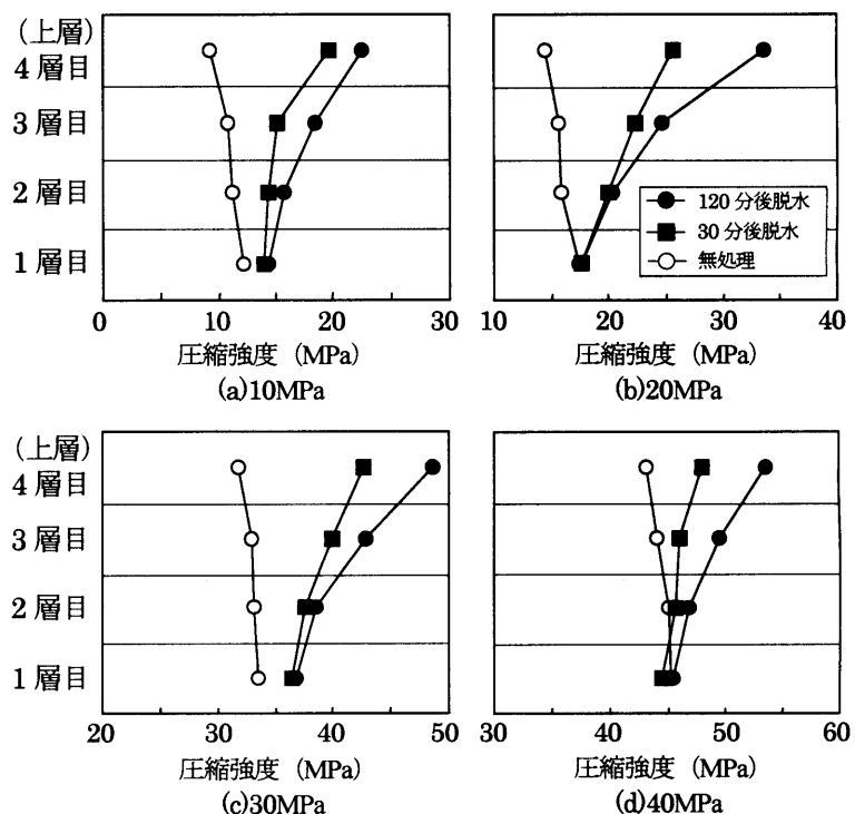
図-8 圧縮強度分布
